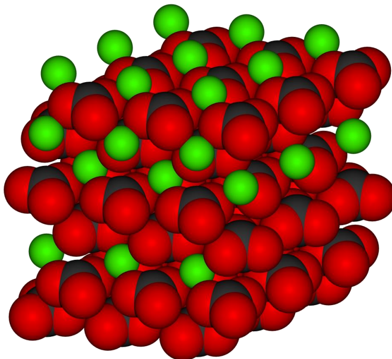
Carbonate de calcium \text{CaCO}_3
