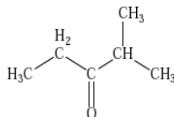
2-méthylpentan-3-one
