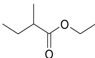
2-méthylbutanoate d'éthyle
