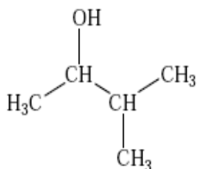
Méthylbutane
