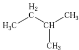
Méthylbutane
