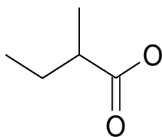
acide 2-méthylbutanoïque
