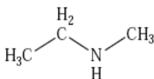
N-méthyléthanimine
