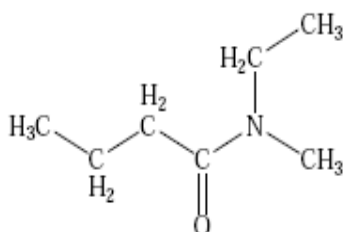
N-éthyl-N-méthylbutanamide
