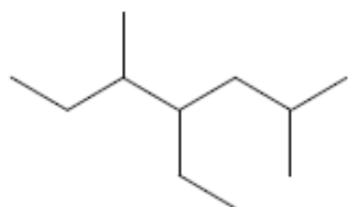
4-éthyl-2,5-diméthylheptane
