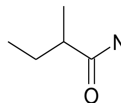
2-méthylbutanamide
