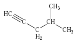
4-méthylpen-1-yne
