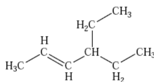
4-éthylhex-2-ène
