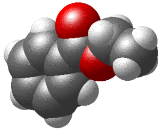
Benzoate d'éthyle
