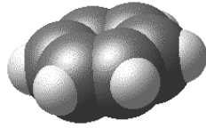
Benzène
