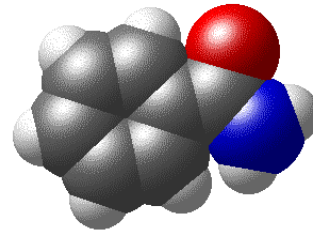
Benzamide
