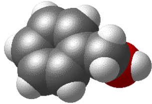
Alcool benzylique
