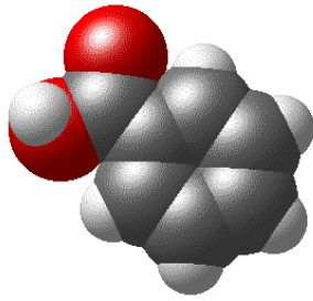
Acide benzoïque
