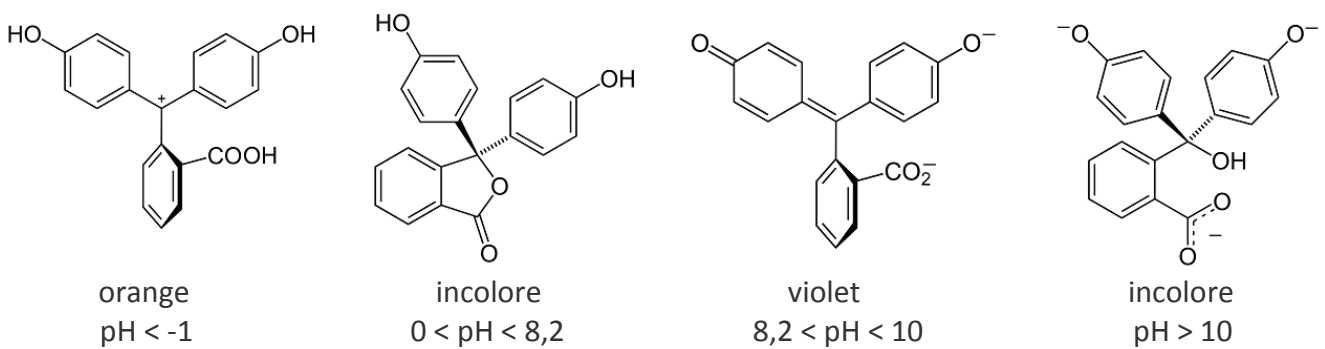
Phénolphaléine [3,3-bis(4-hydroxyphényl)-1-monobenzofuranone]
